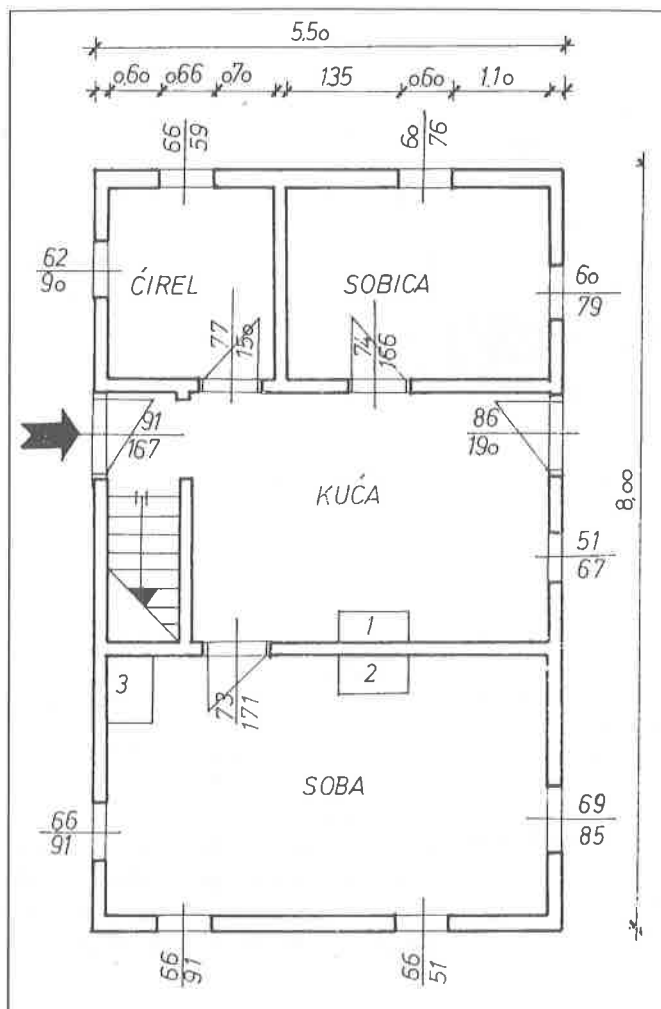
Osnova prizmlja (1. ognjište, 2. furuna, 3. hamamdžik)
