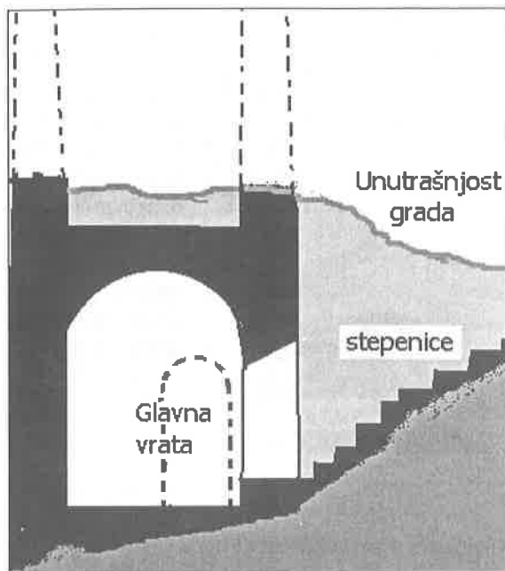
Sl. 6. Ulazna kula - presjek
