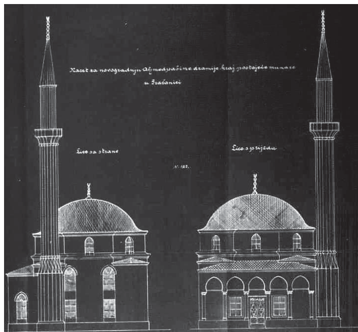
Slika 4. Nacrt za novogradnju Ahmedpašine džamije kraj postojeće munare u Gračanici - Prikaz objekta sprijeda i sa strane
