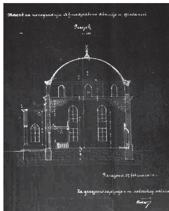
Slika 5. Presjek Ahmedpašine džamije bez munare
